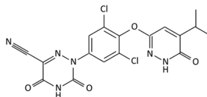
MGL-3196 (Resmetirom)
